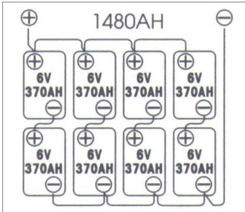
Système 12 volts à 8 batteries 6 volts (mixte)
