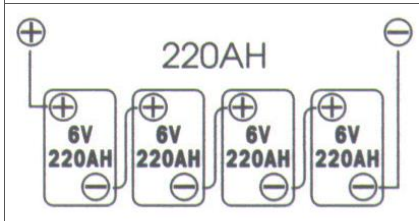
Système 24 volts à 4 batteries 6 volts (en série)
